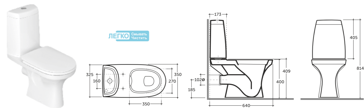
УНИТАЗ-КОМПАКТ САНТИ R WC COMPACT SANTI R
